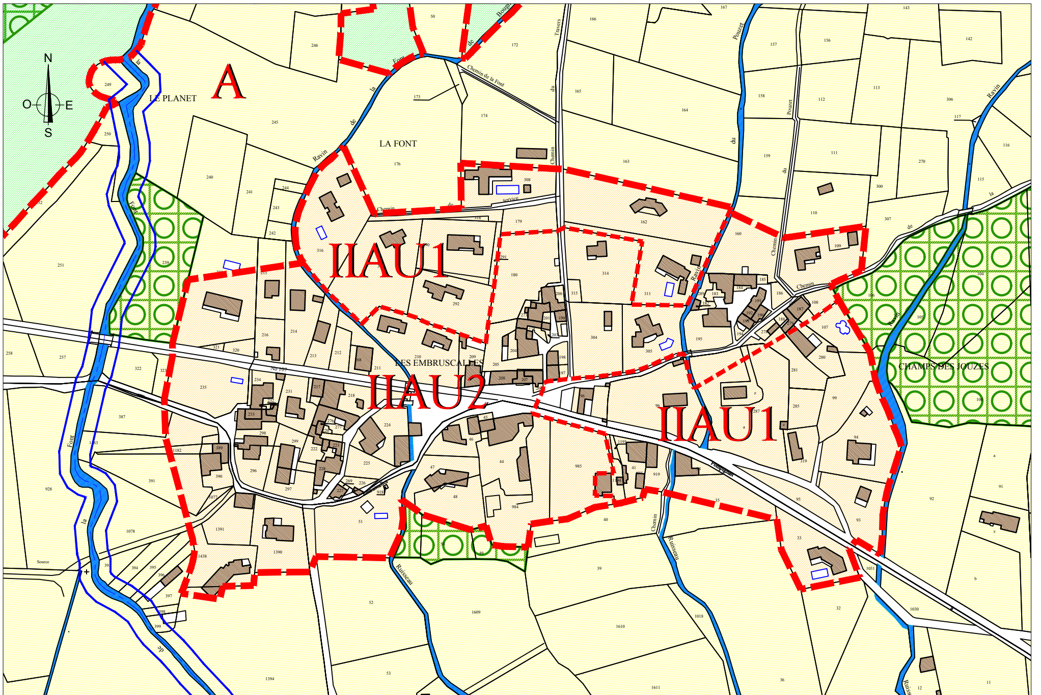
Hameau des Embruscalles - PLU actuellement approuvé - Echelle : 1/2500
